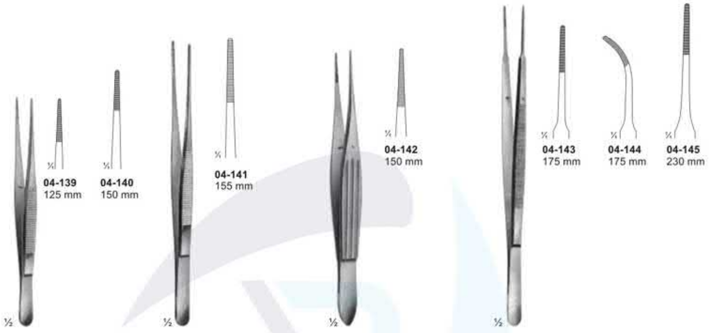
04-139 - 140 SEMKEN
