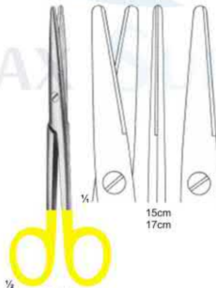
26-111 Mayo-Stille
